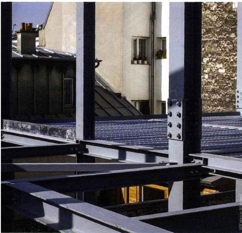
Des planchers en bac acier ont permis de créer très rapidement des plates-formes à chaque étage et ont facilité la construction.
